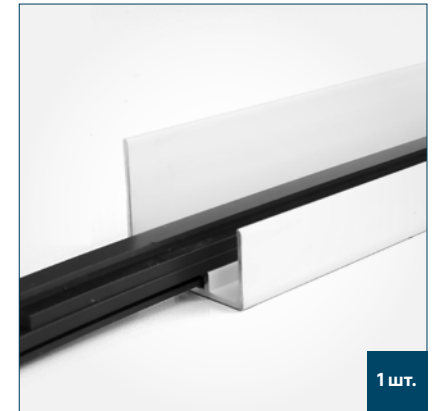
100-00024-XX Направляющая с магнитной полосой 24×22×6000 мм
