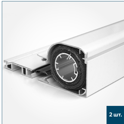
100-01701-XX, 100-11701-XX, 100-02601-XX, 100-12601-XX, 100-21202-XX Кассета в сборе 43×57×6000 мм
