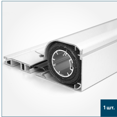
100-01701-XX, 100-11701-XX, 100-02601-XX, 100-12601-XX, 100-21202-XX Кассета в сборе /короб, вал, полотно, тяговая планка/ 43×57×6000 мм
