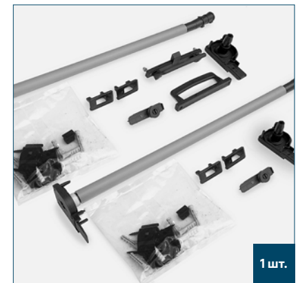
100-00104-05 Комплект для сборки и монтажа
